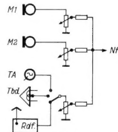
Bild 4. Dreiteiliges Mischfeld mit „Musikeingang“
