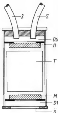
Bild 2. Schnitt durch das Herzschallmikrofon von Ollmann. Ö = Patientenseitige Schallöffnung; D = Druckkammer; T = Raum für Transistorverstärker und Batterie; H = Hörsystem; S = Schallschläuche
