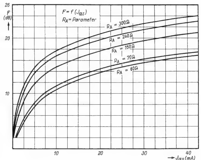
Bild 5a. F = f(I_{as}) ; R_A = \text{Parameter} ; F in dB.
