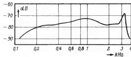
Bild 5. Frequenzkurve des magnetischen Mikrofons M1 Rb für Transistorverstärker
