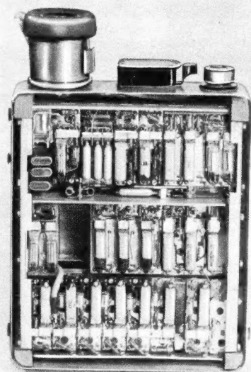
Das neue Telefunken-Kleinfunksprechgerät „Teleport IV“ ist ganz in Subminiaturtechnik ausgeführt. Nicht nur die Röhren, sondern auch alle Bauteile haben entsprechende Größen
