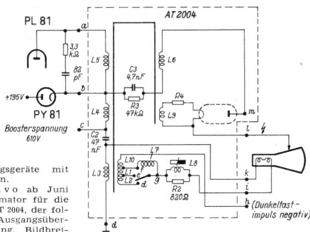
Schaltung des neuen Zeilenausgangstransformators AT 2004 der Valvo GmbH. Primärinduktivität (S1 + S2 + S3 + S4 + S5) = 500 \text{ mH} ; U_a = 16 \text{ kV} bei I_a = 0 ; R_i = 8,3 \text{ M}\Omega
