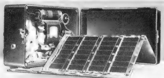
Bild 4. Aus der aufklappbaren Rückwand kann eine dreiteilige Batterie von Fotoelementen herausgeklappt werden
