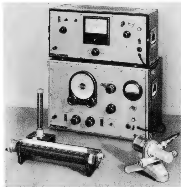
Dämpfungsmeßplatz für 300... 1000 Hz mit dem Siemens-Meßsender 3 W 58
