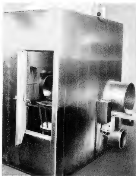
Abschirmkühlig MGL 4100 von Grundig. Die Öffnungen zum Einsteigen, zum Durchschieben der Geräte und zur Belüftung sind vollkommen störstöricher
