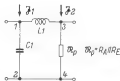
Bild 8. Bestimmung von \mathfrak{I}_2 , der Rauscheinströmung am Empfängereingang. \mathfrak{I}_1 ist die Rauscheinströmung der Rauschdiode für gegebenen Anodenstrom
