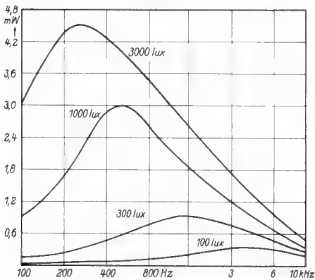
Bild 6. Elektrische Leistung einer Electrocell-Lichtelement-Batterie der Größe 300cm 2 in Abhängigkeit vom Lastwiderstand bei kleinen Beleuchtungsstärken. Das Leistungsmaximum verschiebt sich mit wachsender Beleuchtungsstärke zu kleineren Lastwiderstandswerten. Man erkennt an den Kurven, wie stark die Leistung absinkt, wenn falsch angepaßt wird
