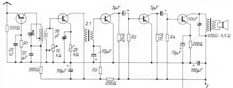
Bild 9. Schaltung des Cellophon II. Die Widerstände R 1 bis R 5 sind vom Transistor-Exemplar stark abhängig, sie sind so zu wählen, daß die aus dem Kennlinienfeld bestimmten Arbeitspunkte eingenommen werden
