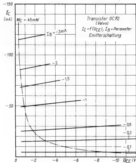
Bild 4. Kennlinienfeld für den Valvo-Transistor OC 72 in Emitterschaltung
