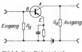
Bild 2. Der Röhrentechniker betrachtet zweckmäßig zuerst nur die Emitterschaltung, um sich mit Transistoren vertraut zu machen; a = Emitterschaltung, b = entsprechende Röhrenschaltung
