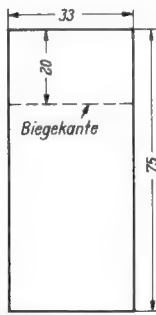
Bild 8. Zuschnitt für die beiden Abschirmbleche
