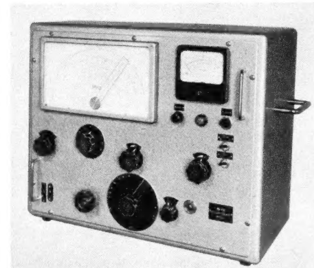
Ein Meßsender für Labor und Prüffeld von der Firma Neuwirth
