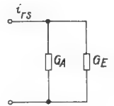
Bild 4. Prinzipschaltung zur Bestimmung der Grenzempfindlichkeit 1/G_A = \text{Antennenstrahlungswiderstand, bzw. für die Rauschmessung der Arbeitswiderstand der Rauschdiode} G_E = \text{Empfängereingangs-Leitwert}
