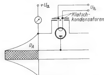
Bild 13. Einbau einer Rauschdiode in eine konzentrische Leitung
