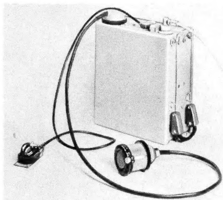
Telefunken-Teleport IV mit Mikrofon/Lautsprecher; links Kanalwahlschalter für getrennte Montage
