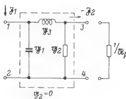
Bild 8a. Umformung von Bild 8 in ein \pi -Glied
