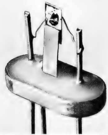
Bild 1. So einfach sieht ein neuzeitlicher Flächen-transistor in starker Vergrößerung aus, und doch ist hierüber eine ganze neue Wissenschaft entstanden (SAF-Transistor ohne Kappe)
