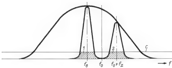
Bild 10. Bei schlechter Spiegelselektion bildet sich im Zf-Verstärker eine höhere Rauschspannung. Sowohl die Rauschfrequenzen von Bereich 1 als auch die von Bereich 2 erzeugen eine Zf-Rauschspannung
