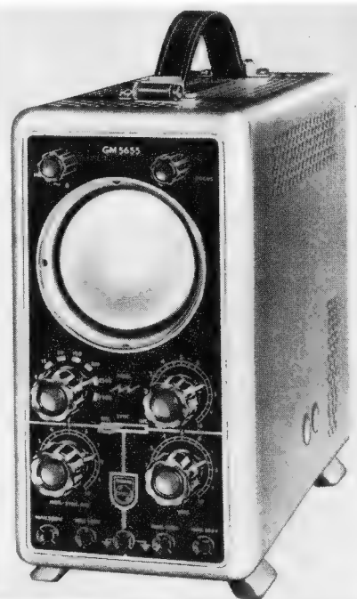
Der handliche Philips-Kleinoszillograf Typ GM 5655/02 mit zwei Meßverstärkern
