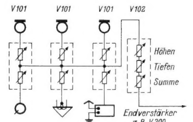
Bild 2. Blockschaltung eines vollständigen Regiefeldes mit Telefunken - Kassettenverstärkern
