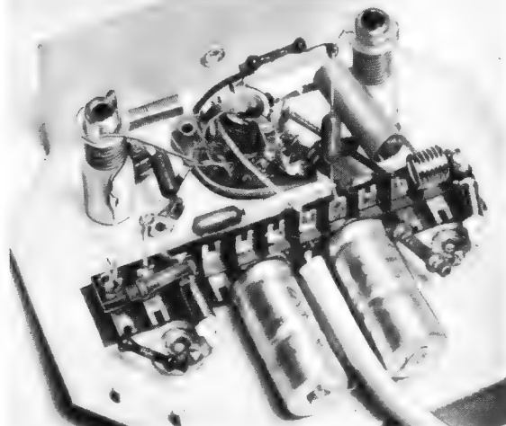
Bild 3. Eingangsschaltung des Empfängers
