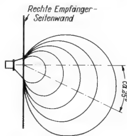
Bild 3. Strahlungsdiagramm des exzentrischen Spezial-Seitenlautsprechers von Isophon
